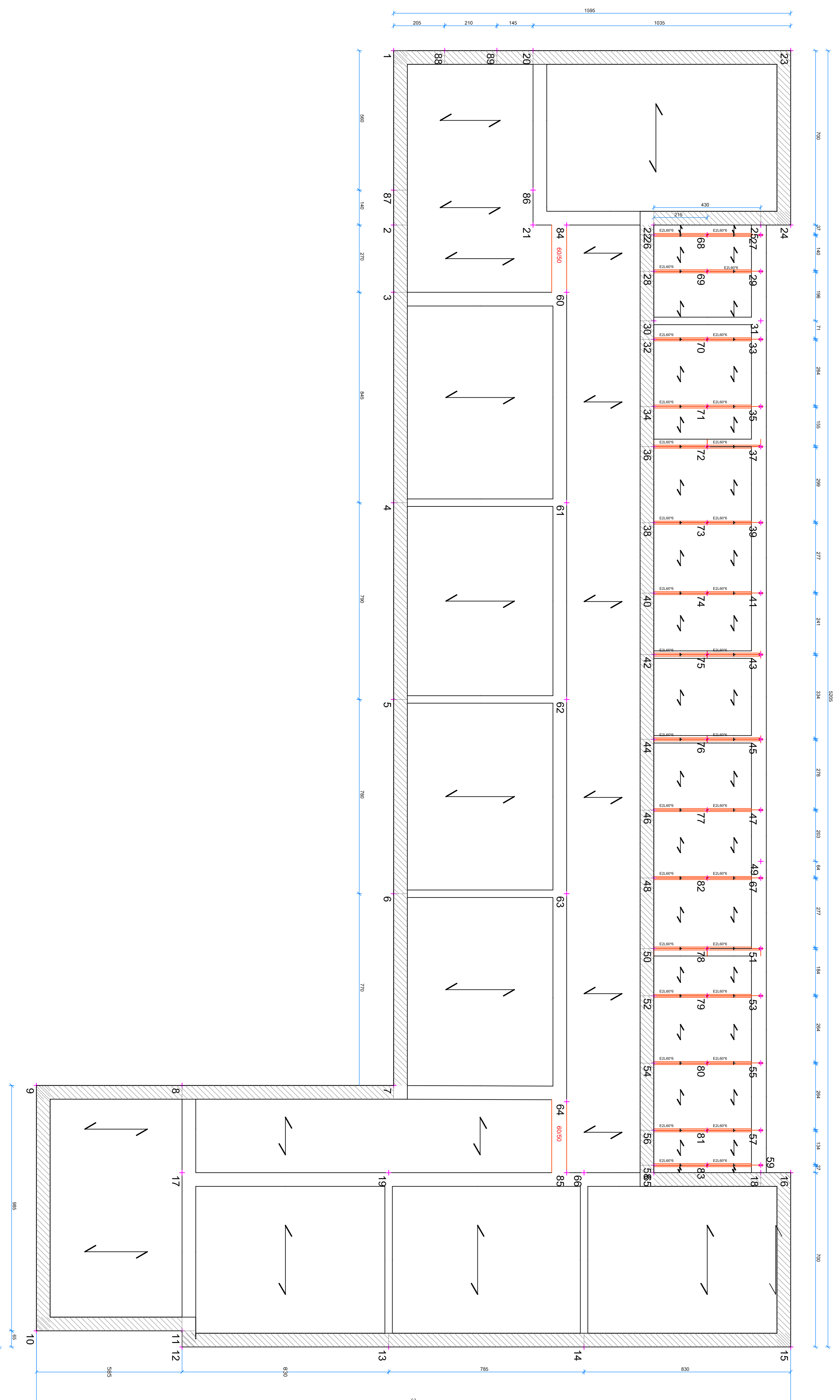
PIANTA IMPALCATO QUOTA m: 7.90 - 2 livello
