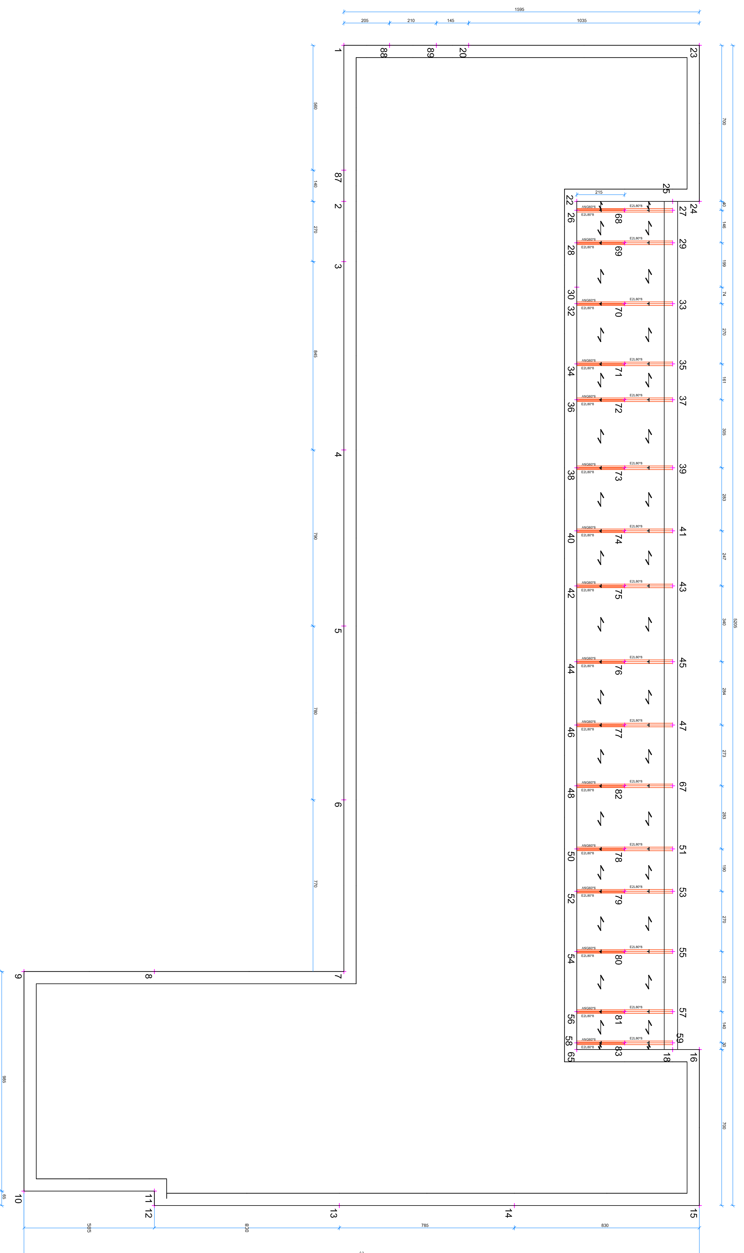
PIANTA IMPALCATO QUOTA m: 9.03 - colmo copertura inclinata
